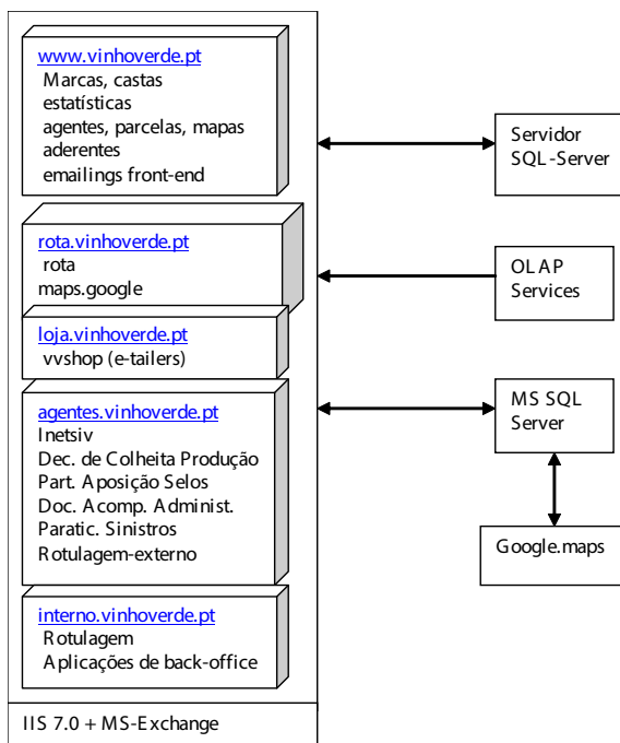
Figura 2: A arquitectura de suporte ao VVRRoute
